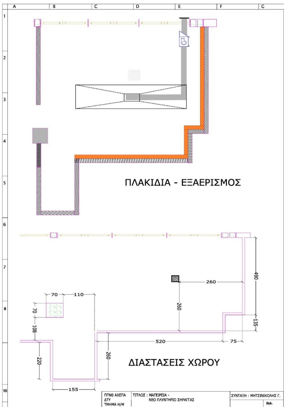
Σχέδιο 3.1: Πλακίδια και εξαερισμός χώρου πλυντηρίου τούνελ
