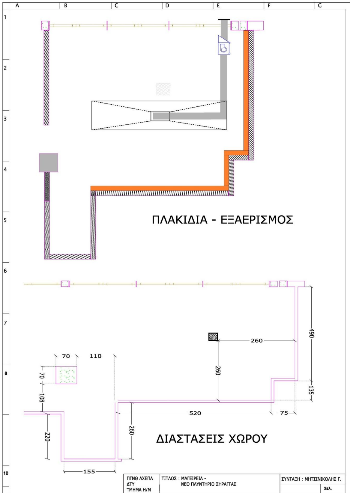
Σχέδιο 3.1: Πλακίδια και εξαερισμός χώρου πλυντηρίου τούνελ
