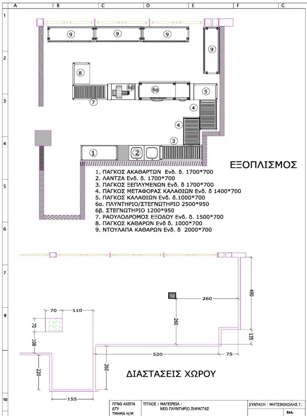
Σχέδιο 3.3: Συνοδος Εξοπλισμός χώρου πλυντηρίου τούνελ.
