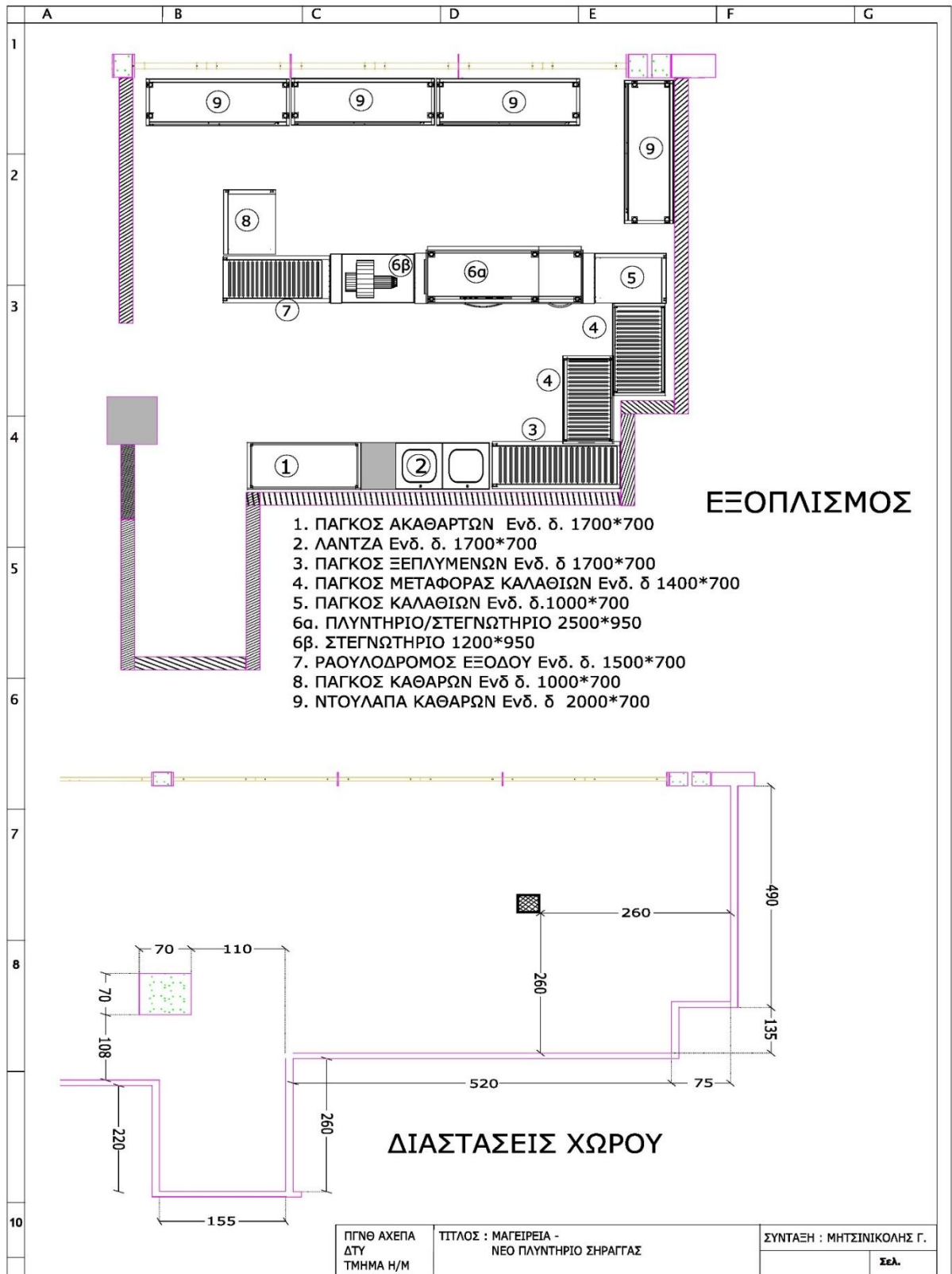
Σχέδιο 3.3: Συνοδος Εξοπλισμός χώρου πλυντηρίου τούνελ.
